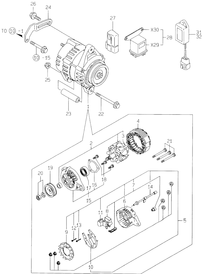
Fig.16. GENERATOR
