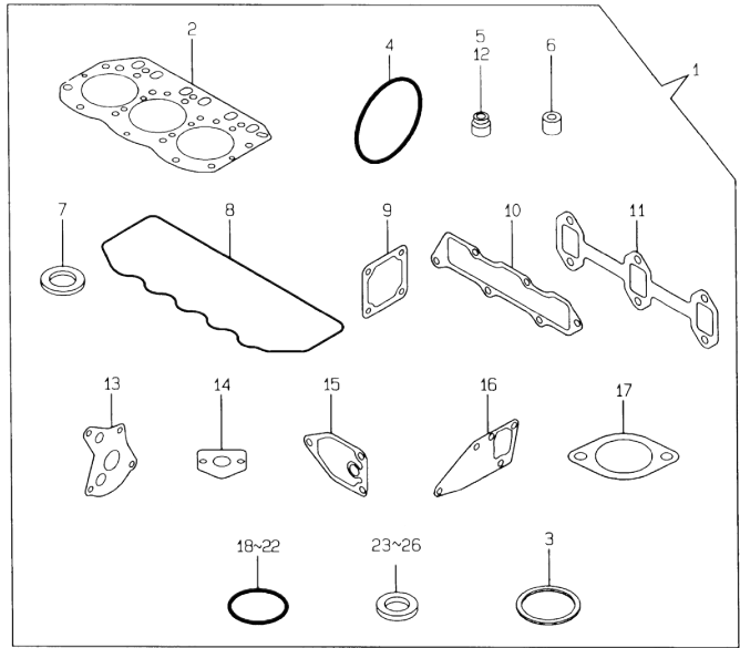
16.GASKET SET
