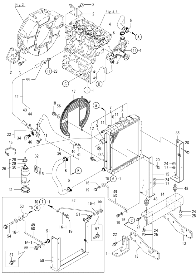
Fig.12. RADIATOR
