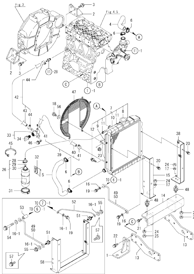
Fig.12. RADIATOR
