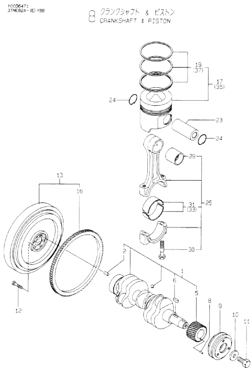
0CD10-M64701 3TNE82A-(E)YBB Fig.8. CRANKSHAFT & PISTON
