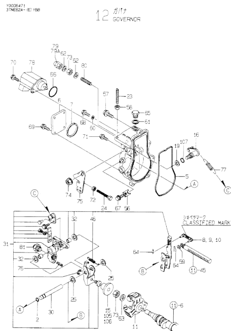
0CD10-M64701 3TNE82A-(E)YBB Fig.12. GOVERNOR
