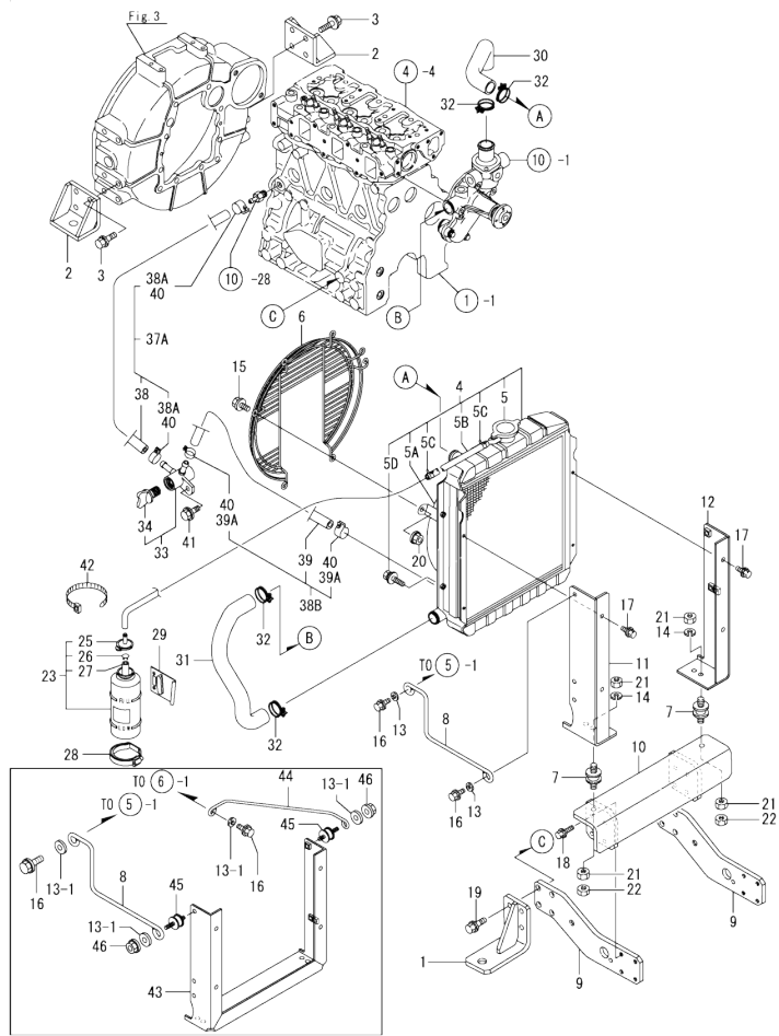
Fig.11. RADIATOR
