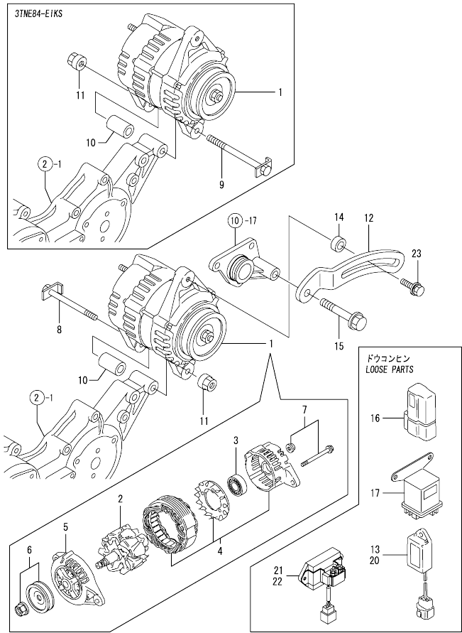
Fig.16. GENERATOR
