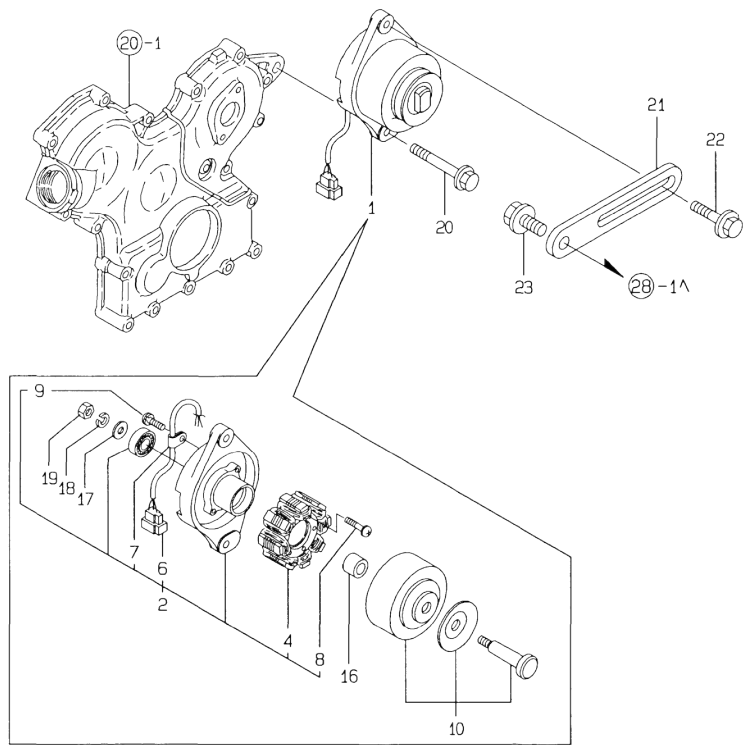
Fig.34. GENERATOR
