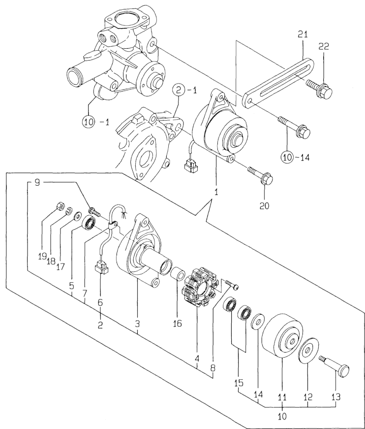
Fig.16. GENERATOR
