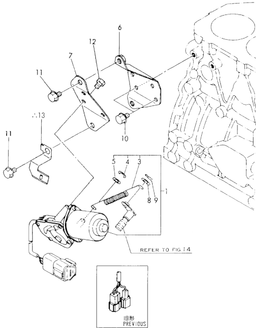
Fig. 15 機関停止装置 ENGINE STOP DEVICE
