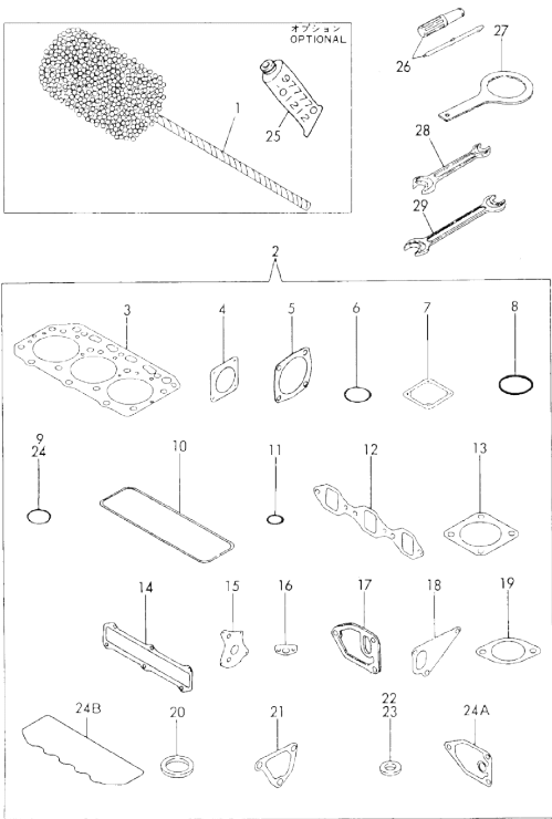
Fig. 18 パッキンセット(オプション)&コウグ GASKET SET (OPTIONAL) & TOOL
