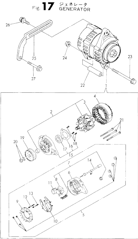
Fig.17. GENERATOR
