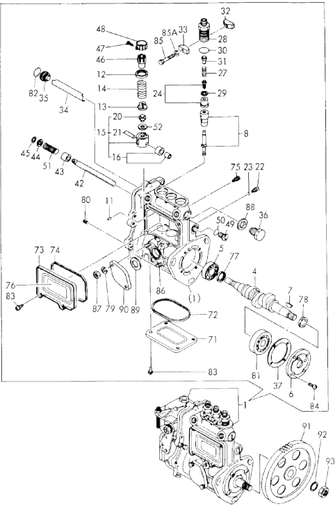
Fig. 11 FOアンシャポンプ FUEL INJECTION PUMP
