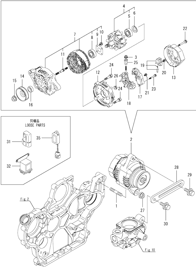
Fig.16. GENERATOR
