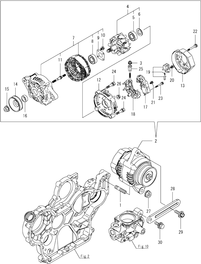
Fig.16. GENERATOR
