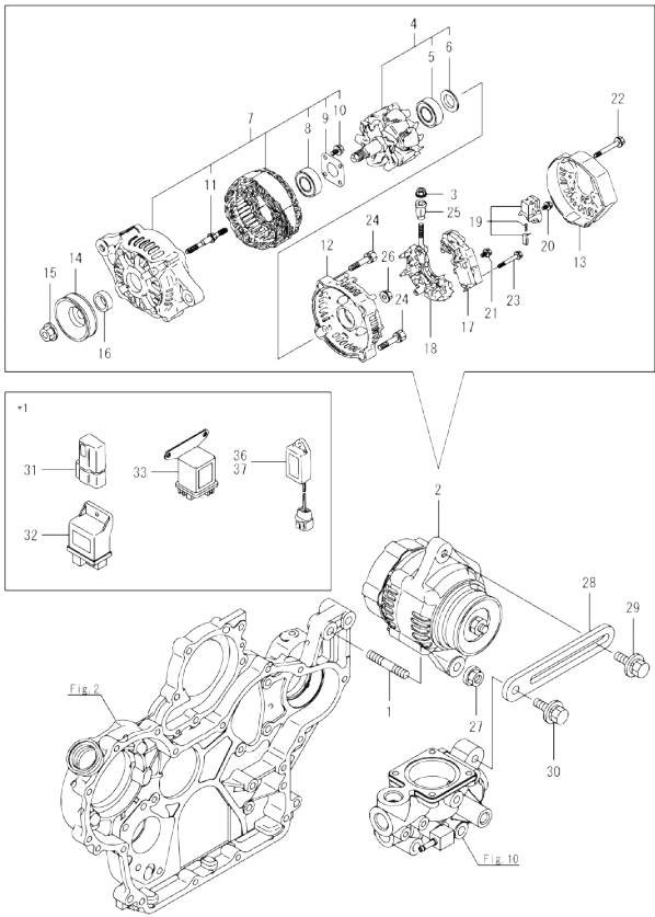
Fig.16. GENERATOR
