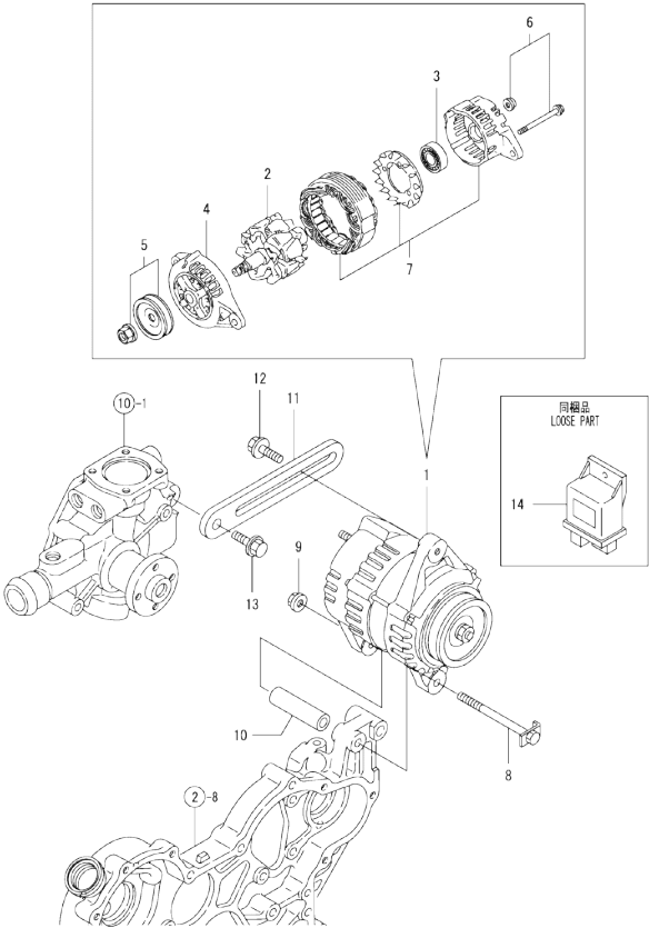
Fig.16. GENERATOR
