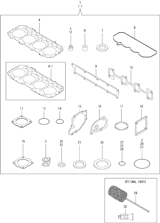
Fig.16. GASKET SET
