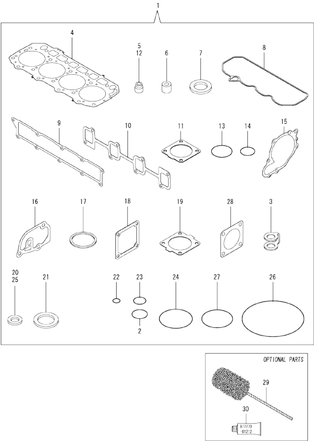
Fig.16. GASKET SET
