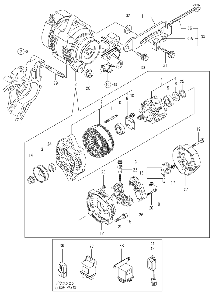
Fig.16. GENERATOR
