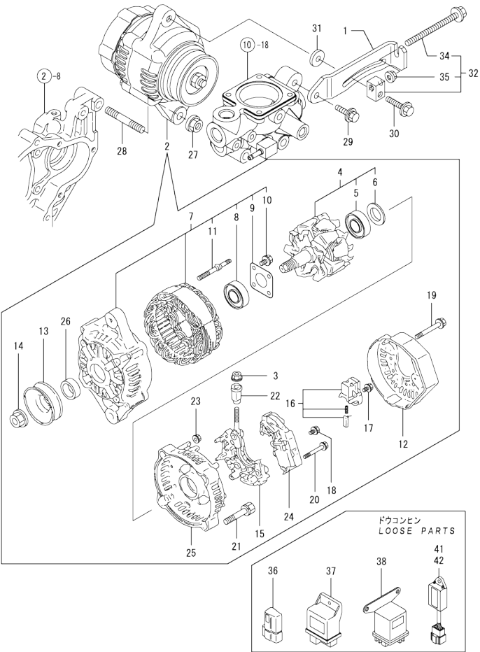
Fig.16. GENERATOR
