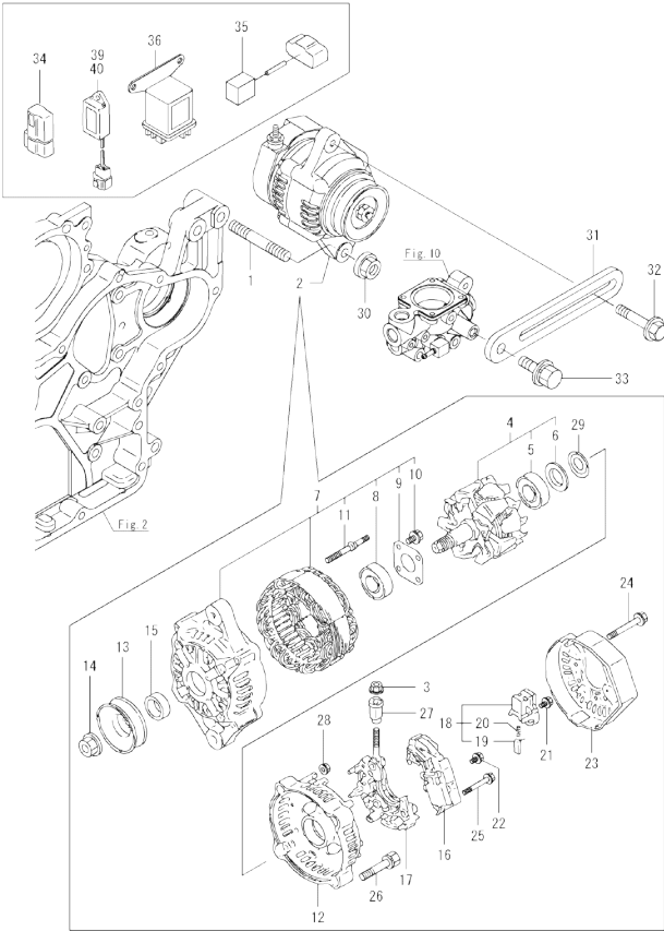
Fig.16. GENERATOR
