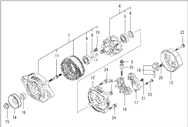
Fig.16. GENERATOR
