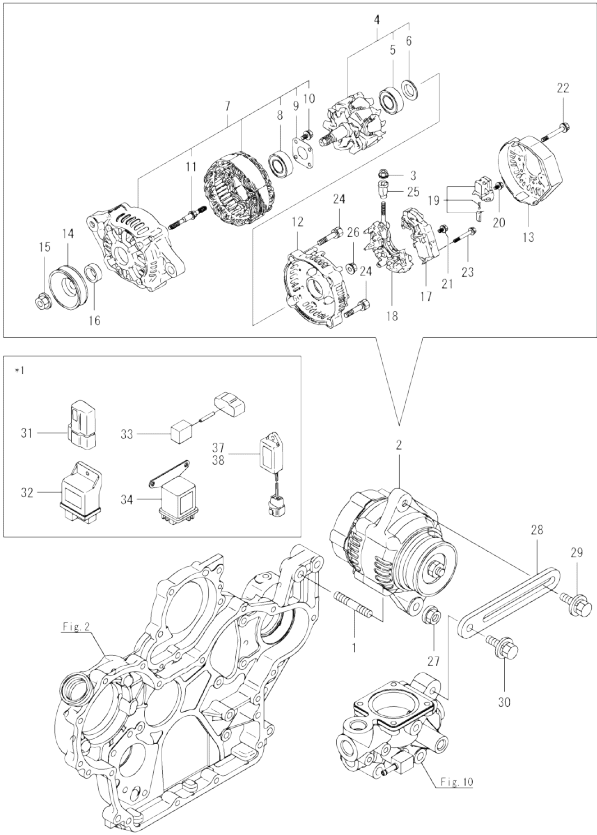
Fig.16. GENERATOR
