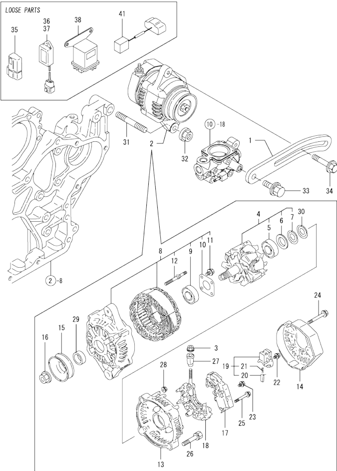
Fig.16. GENERATOR
