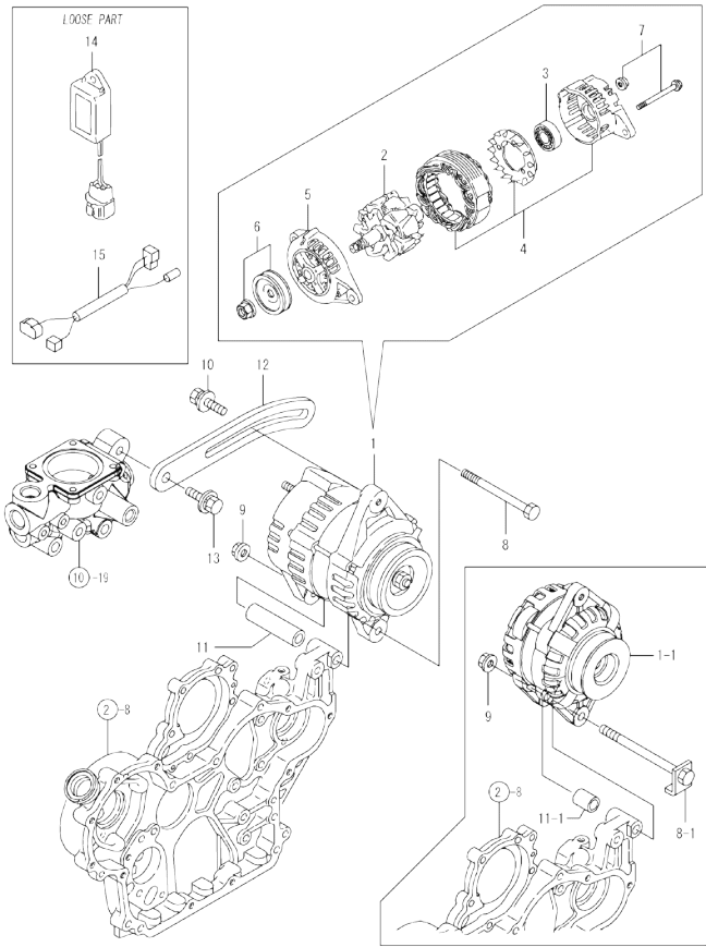
Fig.15. GENERATOR
