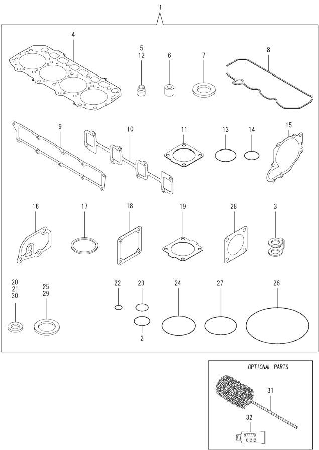
Fig.16. GASKET SET
