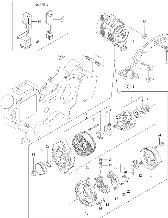
Fig.16. GENERATOR
