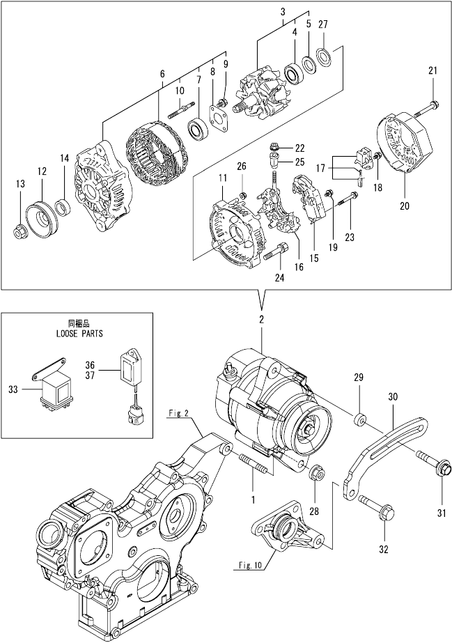
Fig.16. GENERATOR
