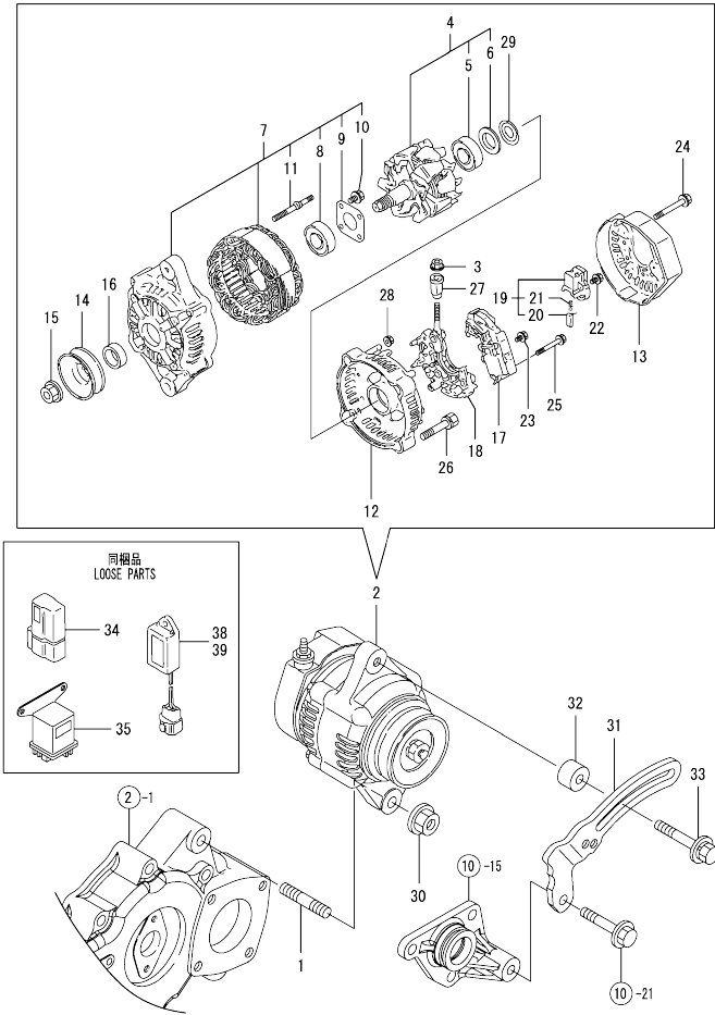
Fig.16. GENERATOR
