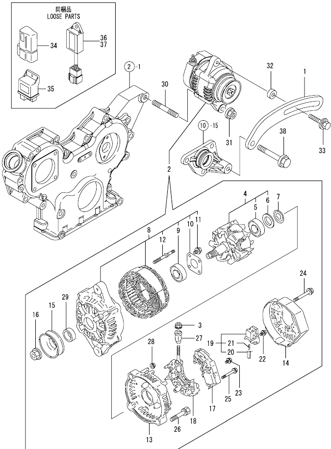
Fig.16. GENERATOR
