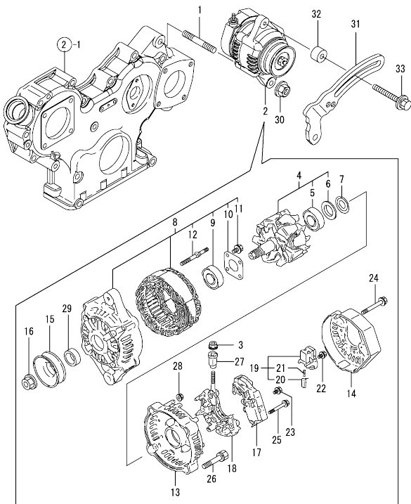
Fig.16. GENERATOR
