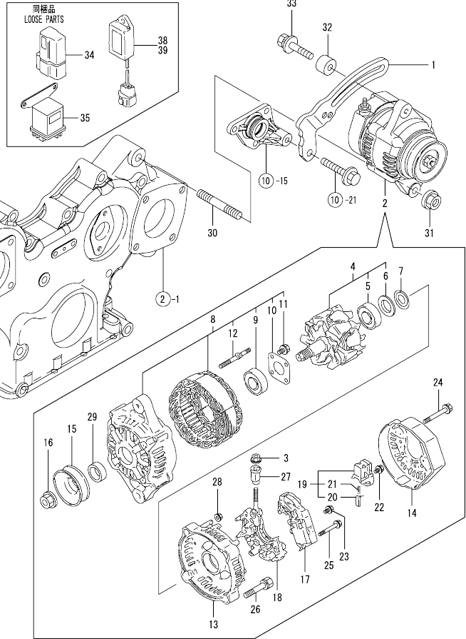
Fig.16. GENERATOR
