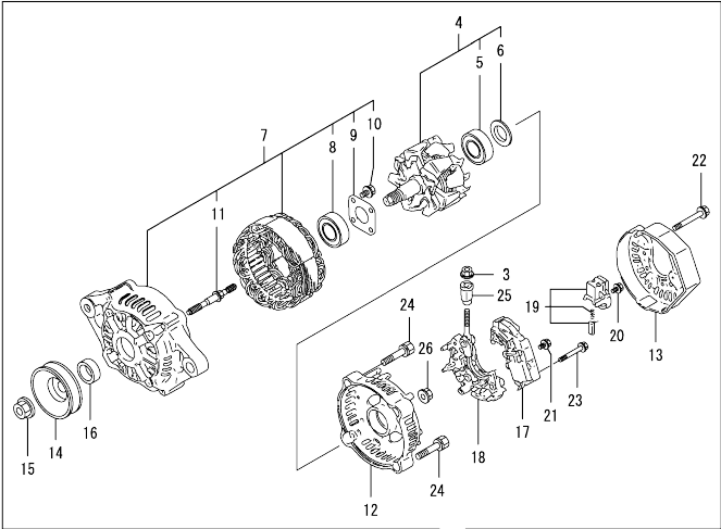
Fig.16. GENERATOR
