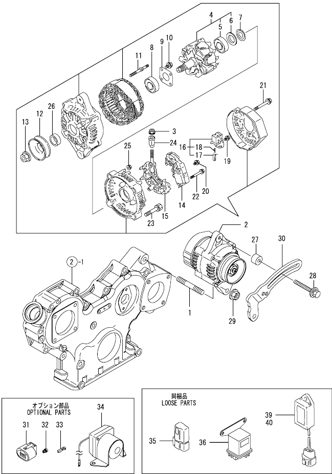
Fig.17. GENERATOR
