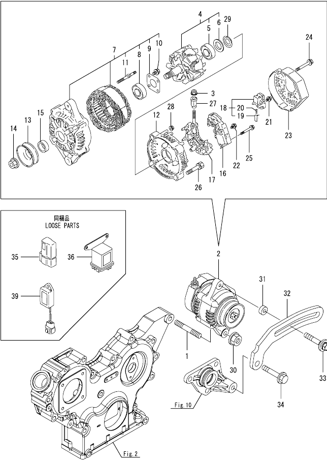
Fig.16. GENERATOR
