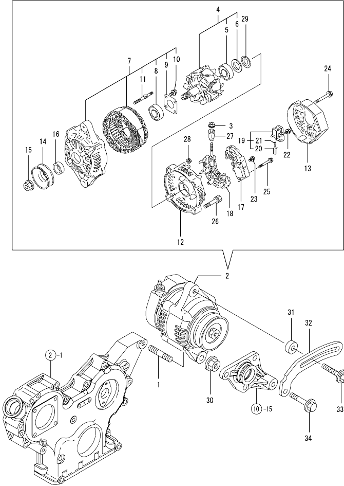
Fig.16. GENERATOR
