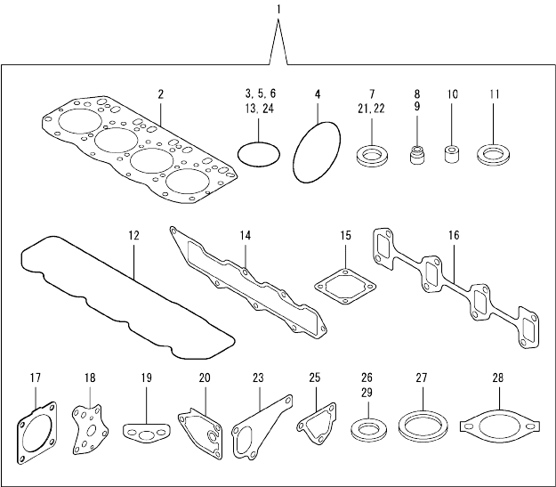
Fig.34. GASKET SET
