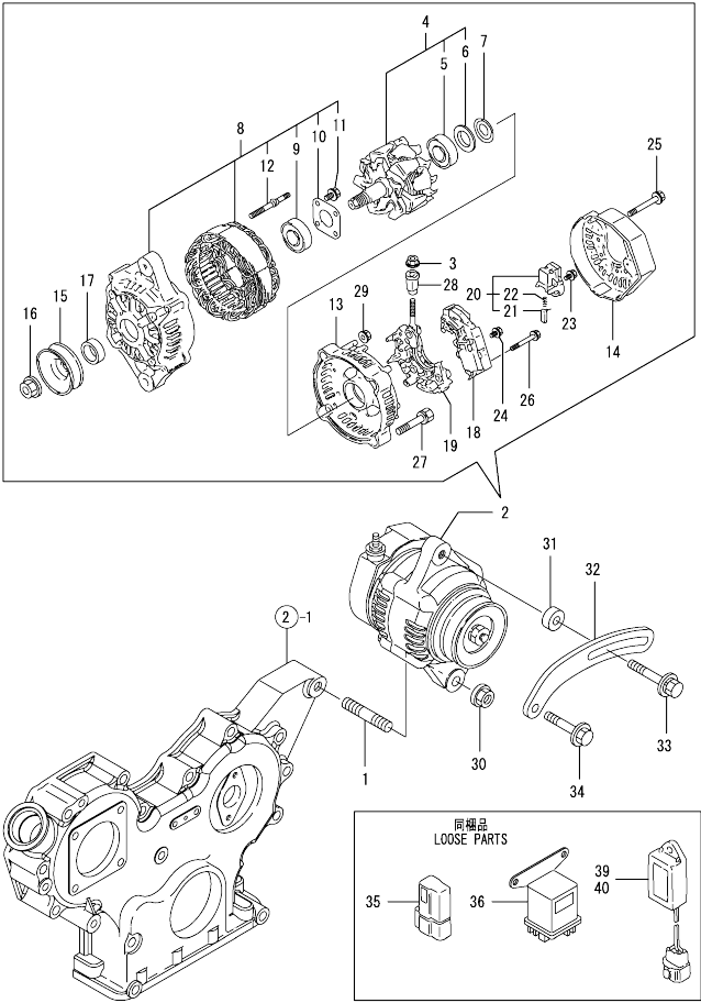
Fig.16. GENERATOR
