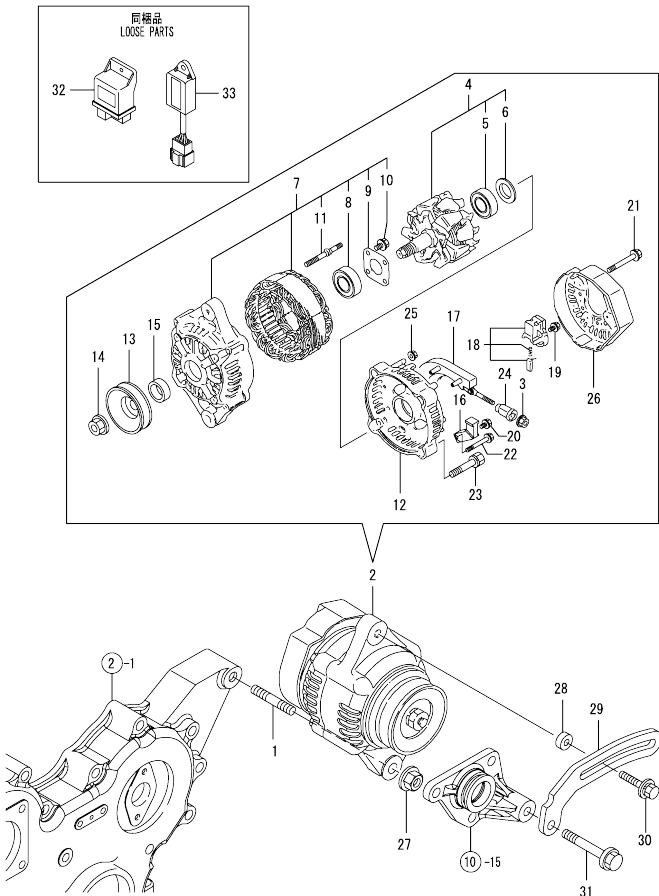
Fig.16. GENERATOR
