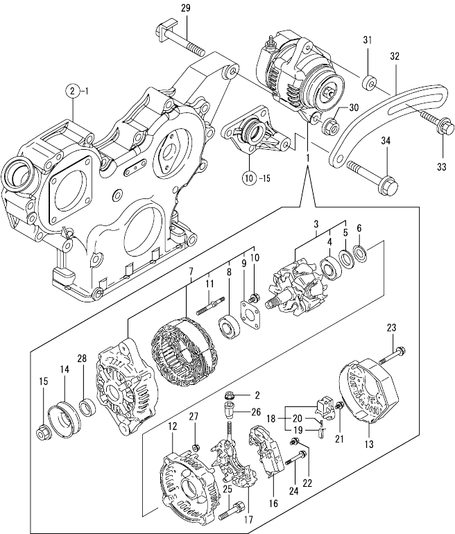
Fig.16. GENERATOR
