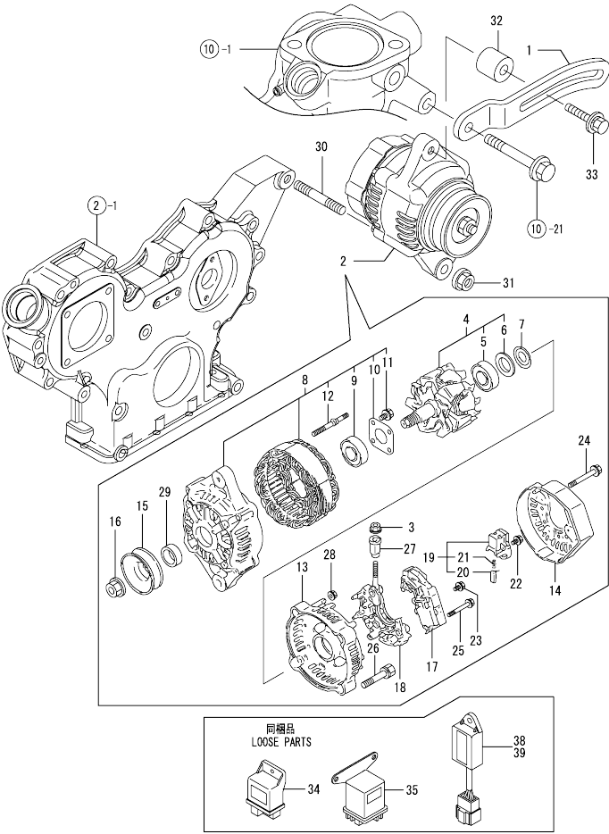
Fig.16. GENERATOR
