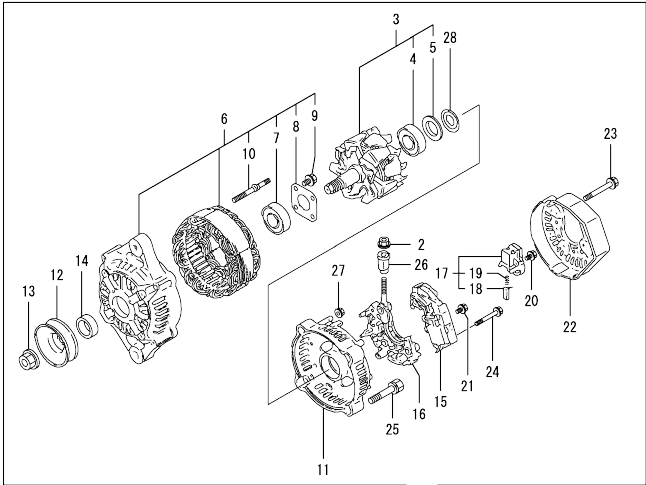
Fig.16. GENERATOR
