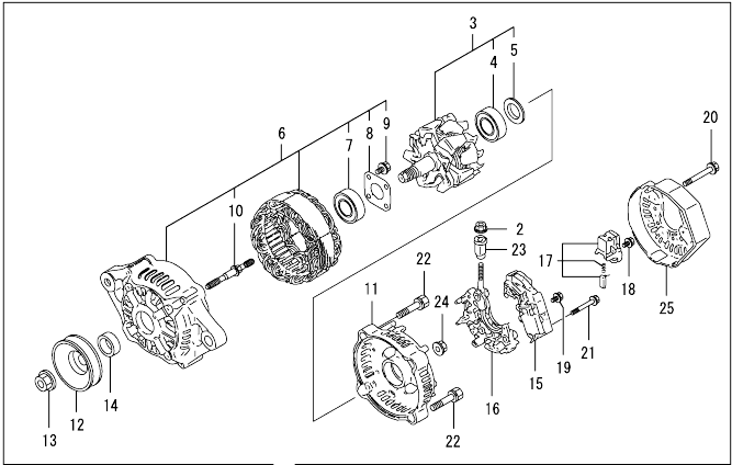
Fig.16. GENERATOR
