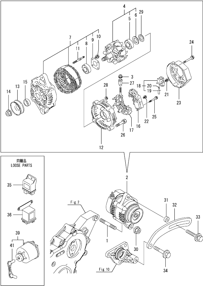
Fig.16. GENERATOR
