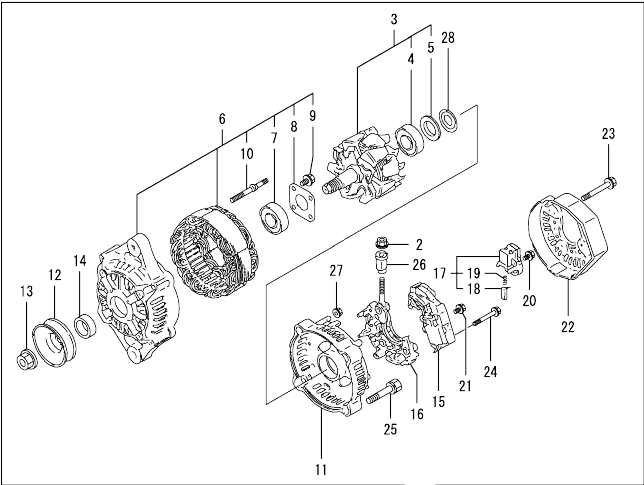
Fig.16. GENERATOR
