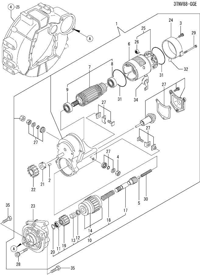
Fig.16. STARTER MOTOR
