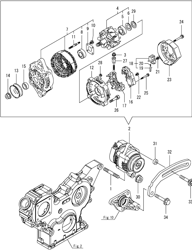
Fig.16. GENERATOR
