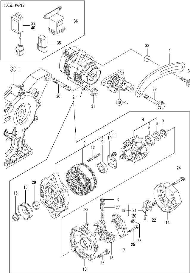
Fig.16. GENERATOR
