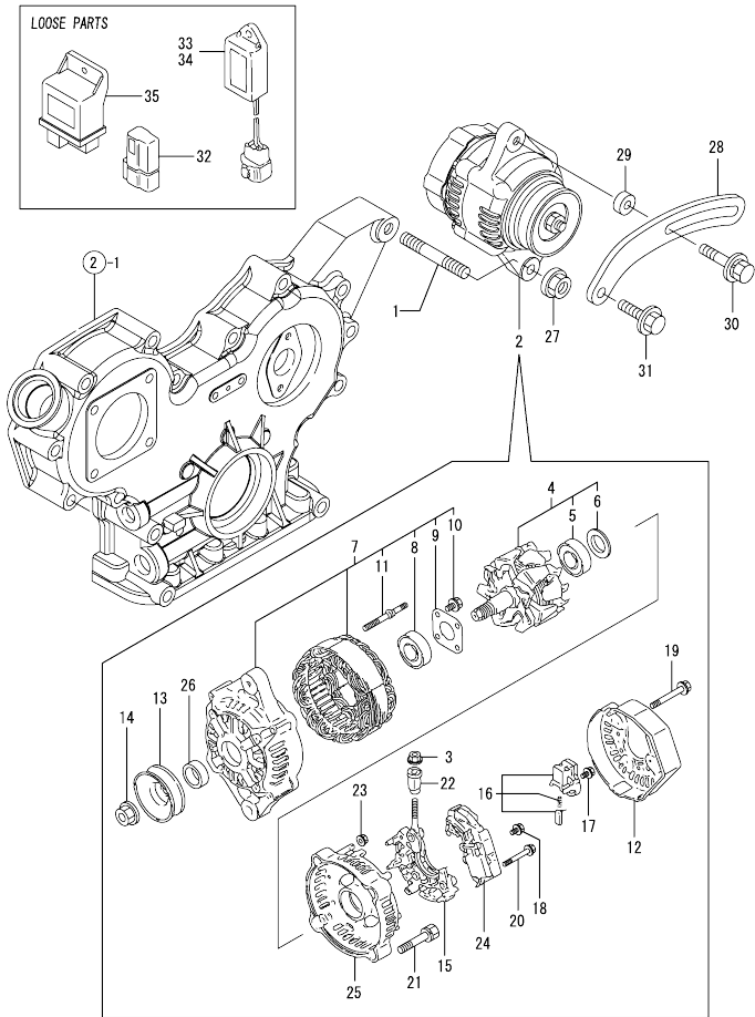
Fig.16. GENERATOR
