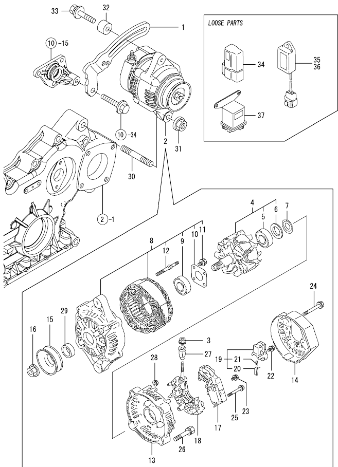
Fig.16. GENERATOR
