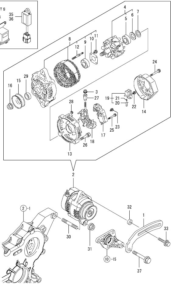
Fig.16. GENERATOR
