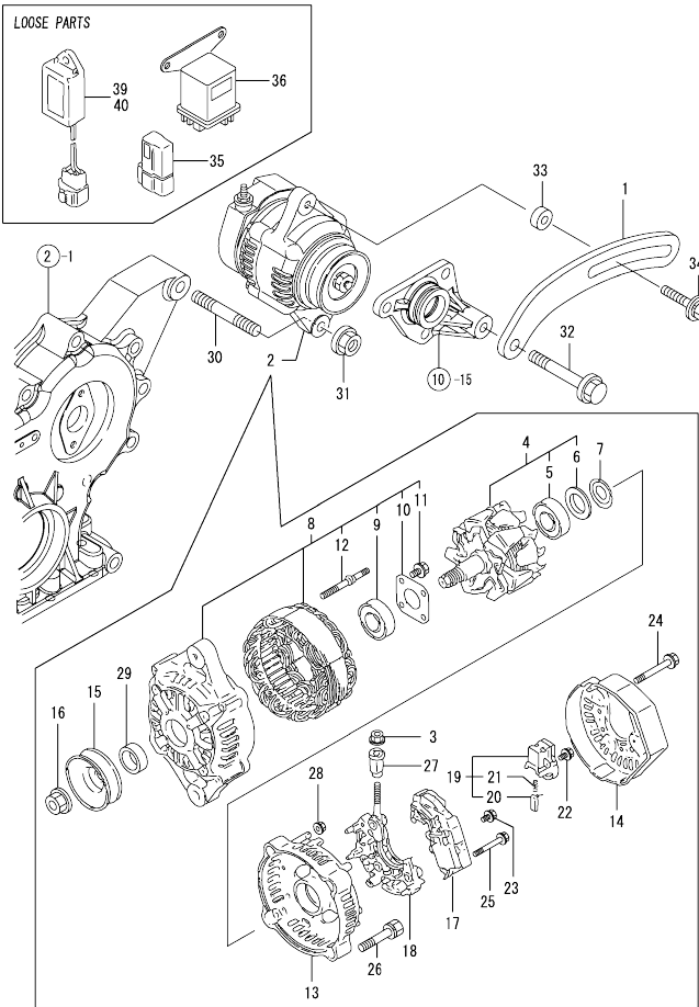
Fig.15. GENERATOR
