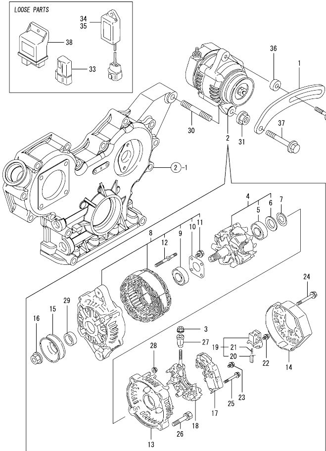
Fig.16. GENERATOR
